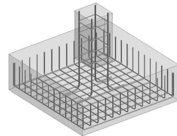
4 3D – výztuž patky P1
