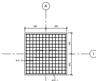
1 Tvary výztuže 1 : 25
