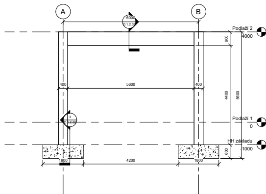
Řez 1-1 – tvar rámu
