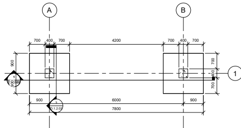
Půdorys základů – tvar
